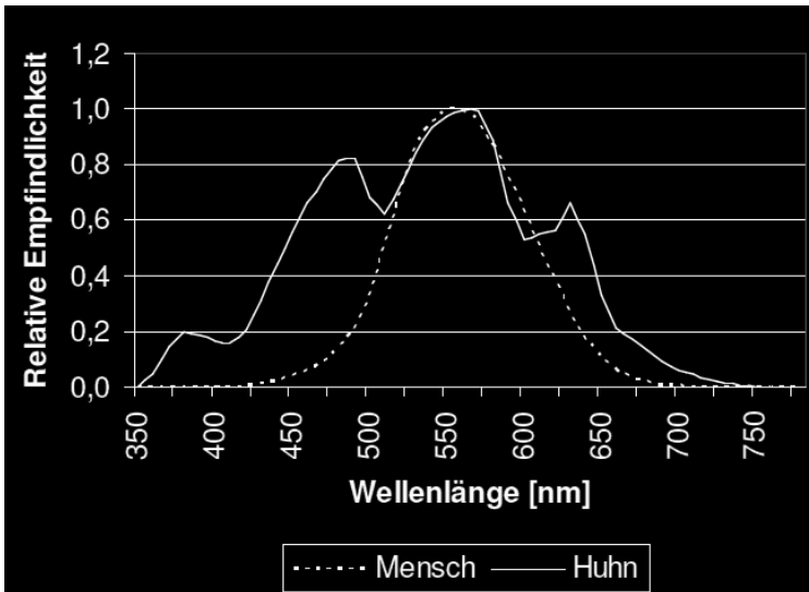
Abbildung 1: Spektrale Empfindlichkeiten von Mensch und Huhn (Aus Weise, Heinrich 2007)
