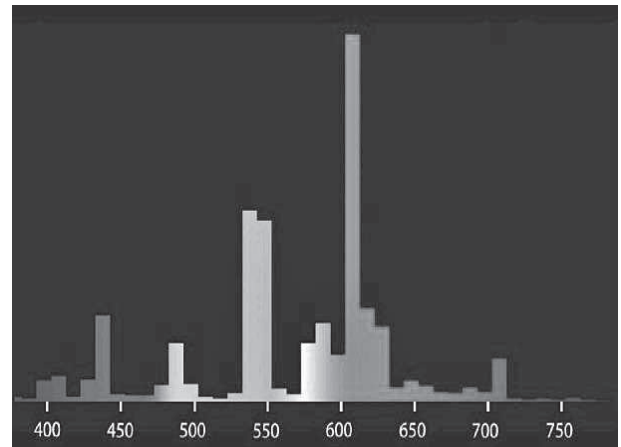
Farbspektrum/ Wellenlänge [nm]: Osram T8 „Biolux“ / Osram T8 „warm-weiss“
